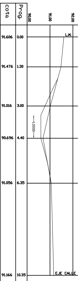
PERFIL PROGRESIVA 1800 MARIA TERESA DE CALCUTA
